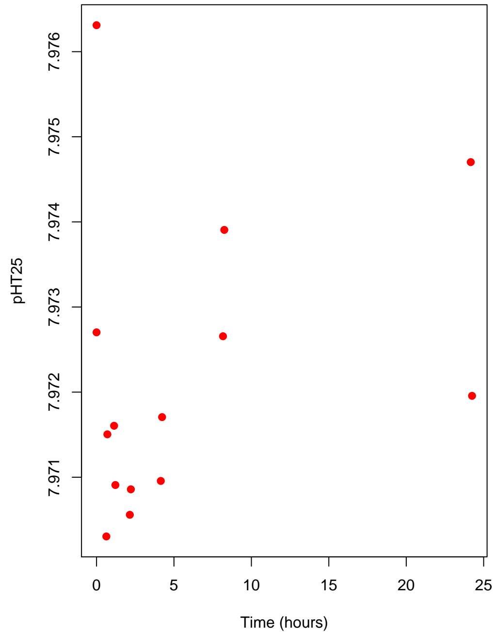
cinetique au cast 77, niskin 4 ( 5 dbar)
