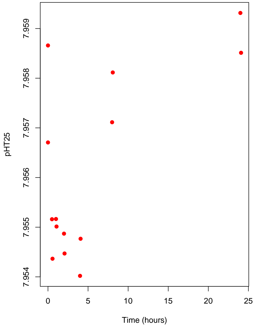
cinetique au cast 77, niskin 2 ( 1500 dbar)
